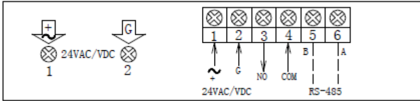
Figure.3 Wiring
